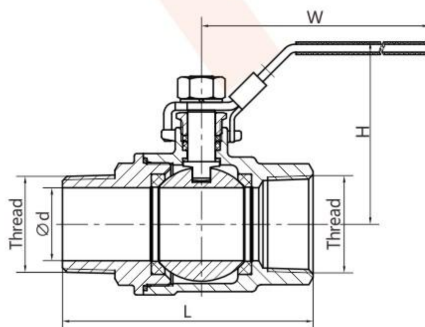
一端内螺纹 一端外螺纹
